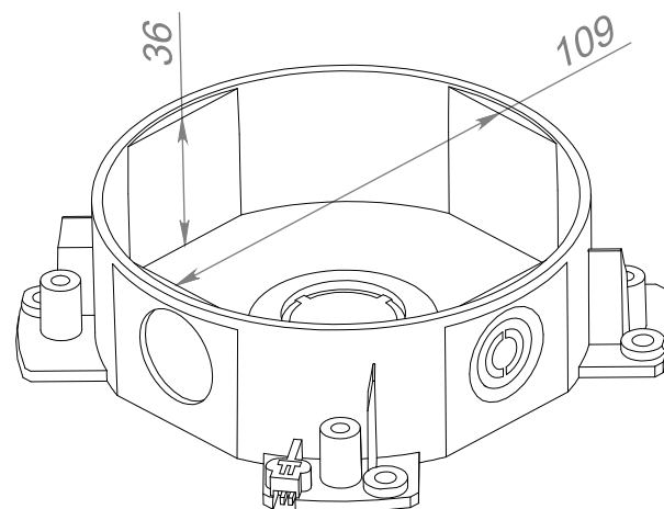
МОНТАЖНАЯ КОРОБКА МК-3, МК-3 ПРО ГАБАРИТНЫЕ И УСТАНОВОЧНЫЕ РАЗМЕРЫ
